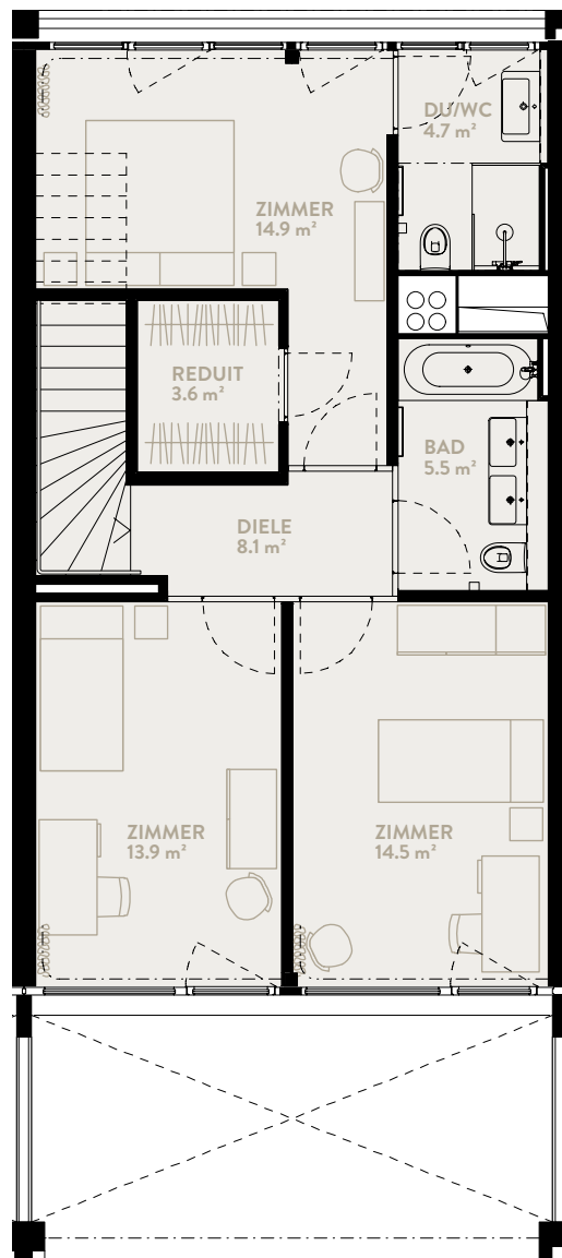
OBERES GESCHOSS
