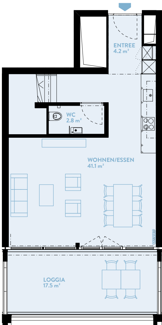
UNTERES GESCHOSS
