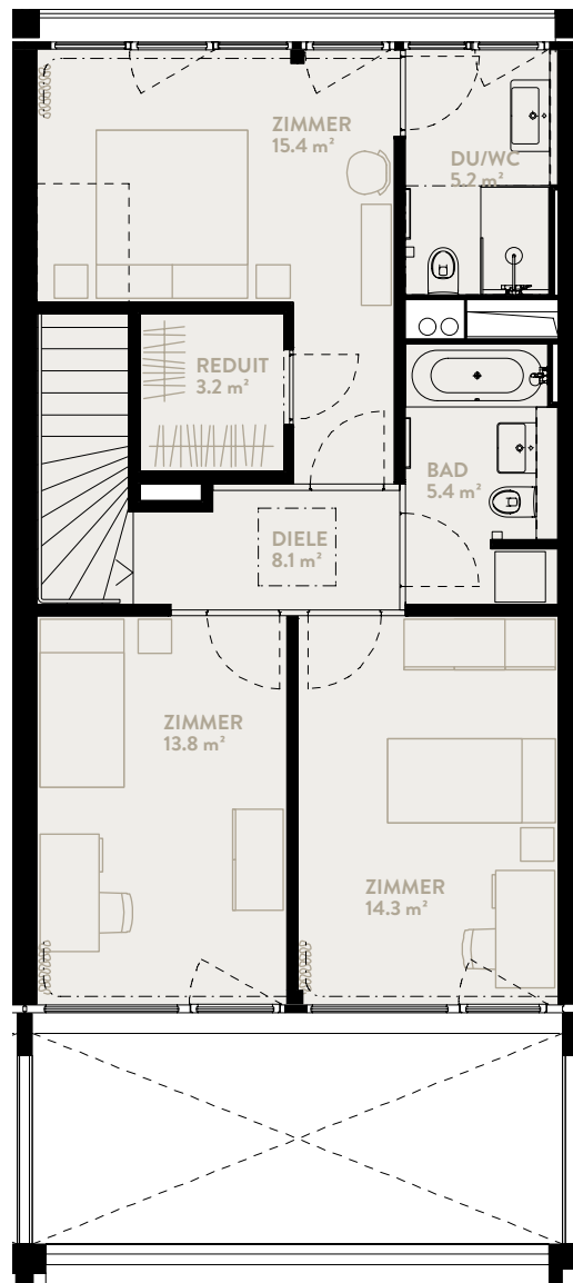
OBERES GESCHOSS
