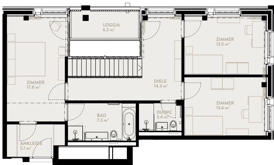
2. MAISONNETTE-GESCHOSS
