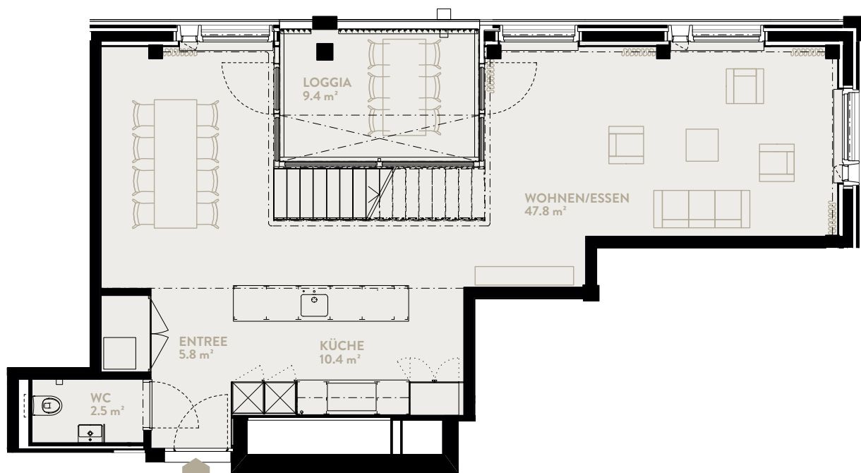
1. MAISONNETTE-GESCHOSS
