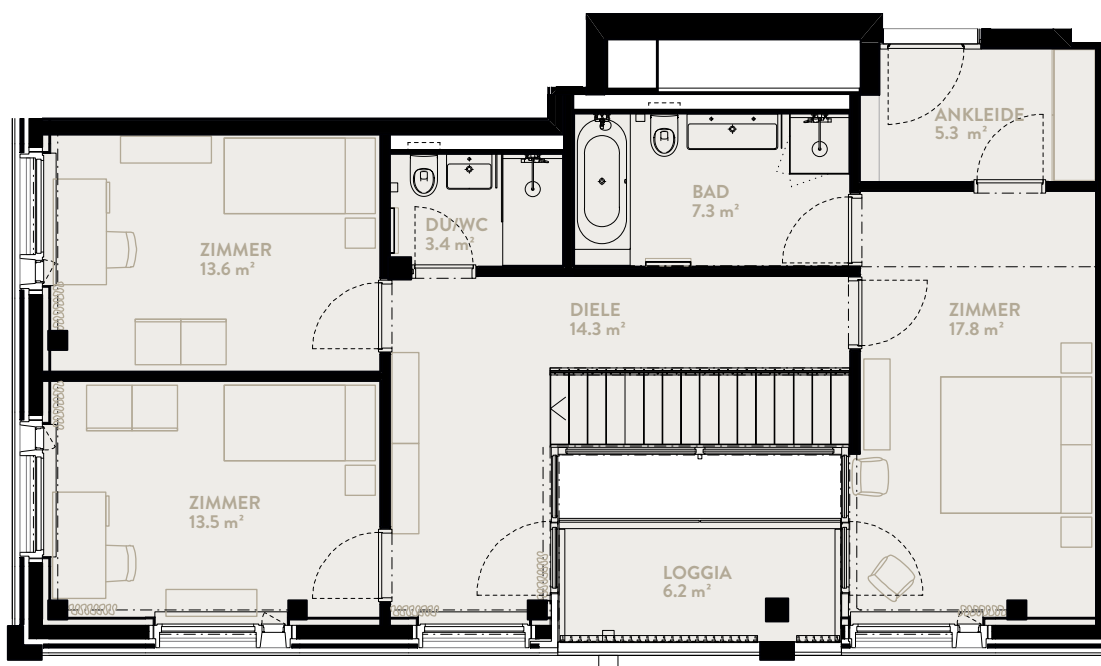
2. MAISONNETTE-GESCHOSS
